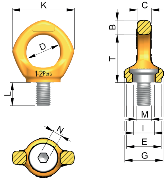
Imagen. 3: Dibujo acotado PSA INOX-STAR para 1-2 personas
