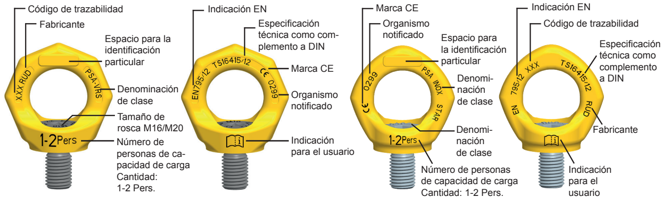
PSA VRS para 1-2 personas
