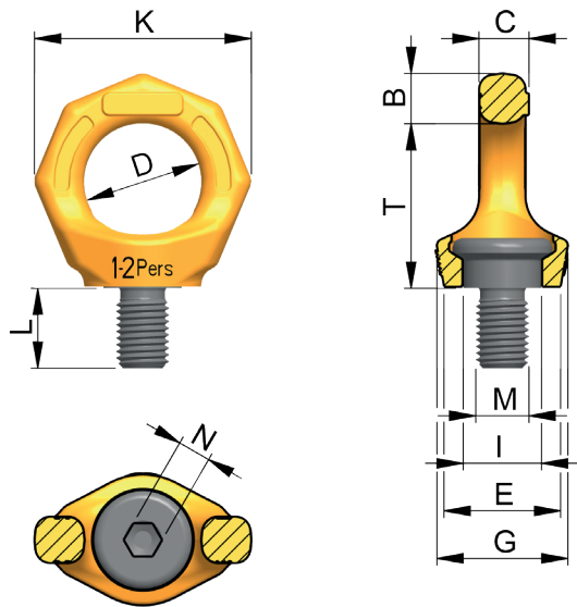
Imagen. 2: Dibujo acotado PSA VRS para 1-2 personas
