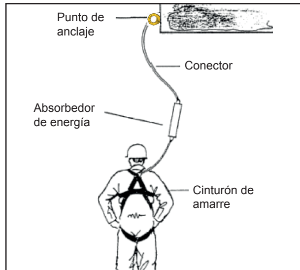
Imagen. 1: Vista general de un sistema de retención con absorbedor de energía (fuente: BGR/GUV-R 198, 03/2011, v. 13 imagen 7)
